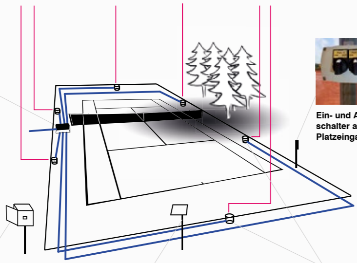
Schacht mit Hauptzuleitung und Magnetventilen
